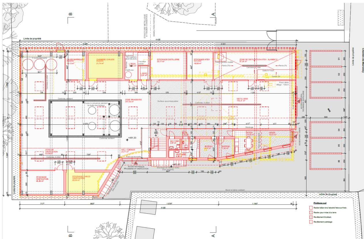
Plan du rez-de-chaussée déposé à l'OAC pour demande d'autorisation de construire initiale
