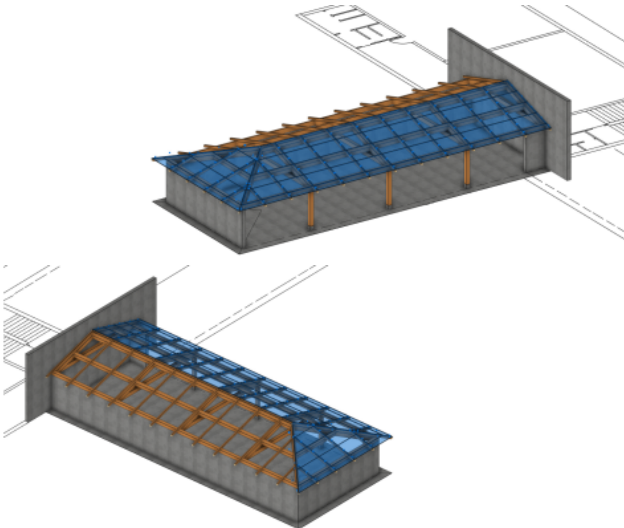
Modélisation 3D du principe constructif (source Charpente Concept)
