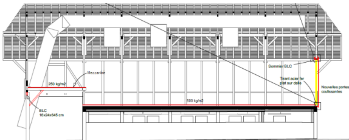
Coupe longitudinale
